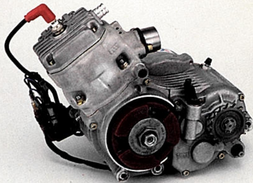
MOTORE KART 125 C-1-C INTERNAZIONALE
