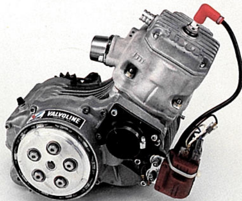
MOTORE KART 125 C NAZIONALE LAMELLARE
