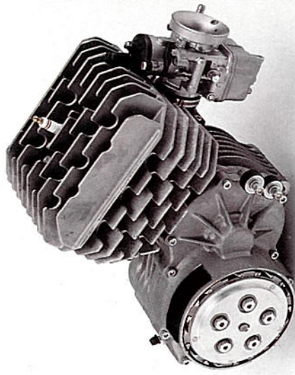
MOTORE KART 125 CATEGORIA NAZIONALE
